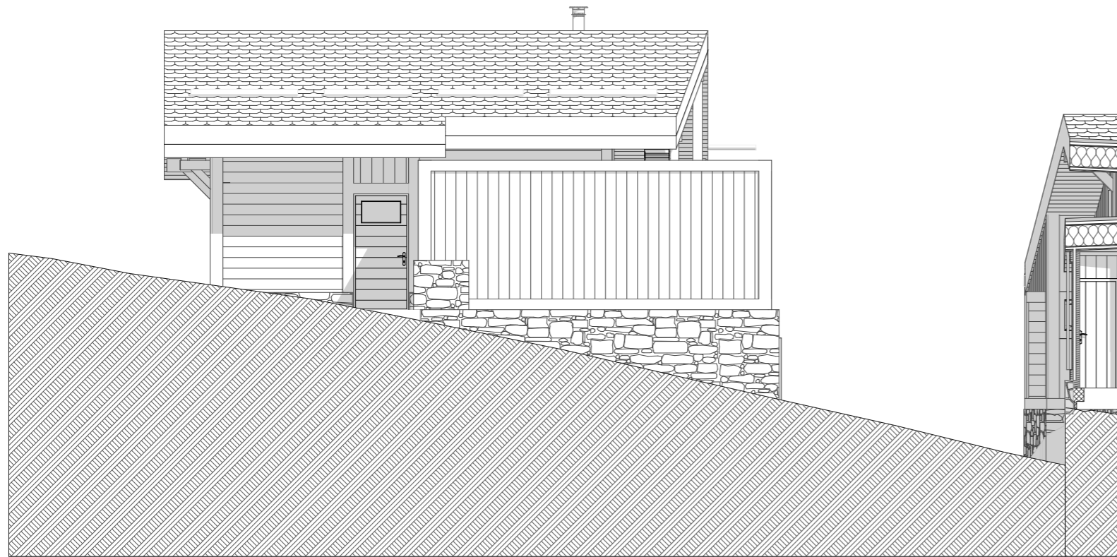
Façade Sud-Ouest
